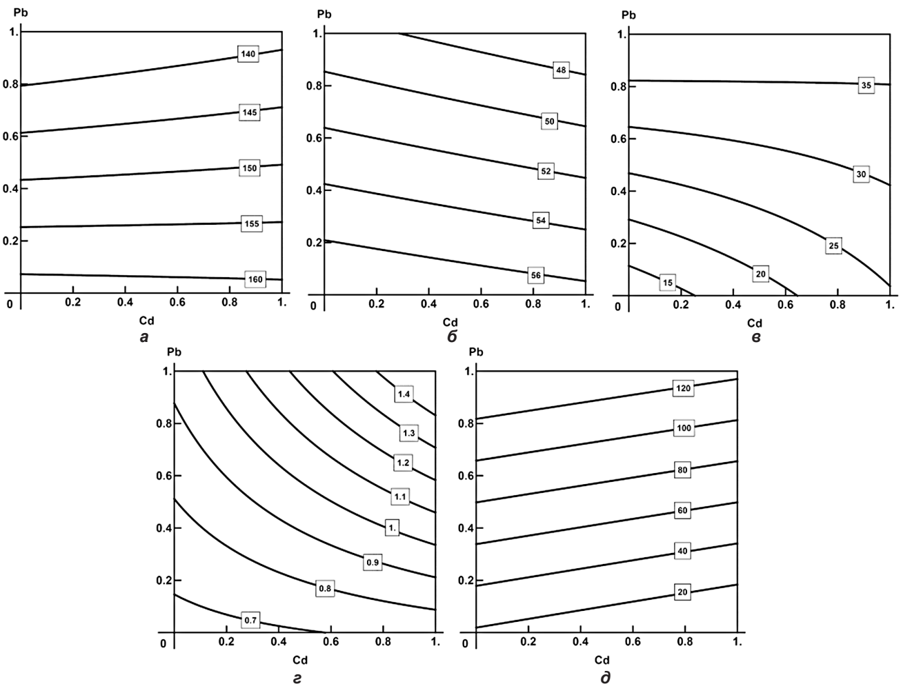
Рис. 3. Примеры изоболограмм, иллюстрирующие неоднозначность типа комбинированного действия кадмия (Cd) и свинца (Pb) на различные показатели состояния организма: а – содержание гемоглобина в крови (преимущественно однофакторный эффект свинца); б – гематокрит (аддитивность однонаправленного действия); в – пропорция ретикулоцитов (субаддитивность однонаправленного действия с переходом при более высоких дозах свинца в его однофакторный эффект); г – число моноцитов (супераддитивность однонаправленного действия с переходом при более высоких дозах свинца и кадмия в аддитивность); д – содержание \delta -АЛК в моче (противонаправленность действию).
